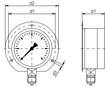
Typ R10.U.3.N...
