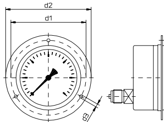
Typ R10.H.2.N...
