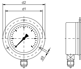
Typ R10.U.2.N...
