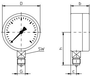
Typ R10.U.1.N...
