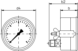
Typ R10.H.4.N... *)
