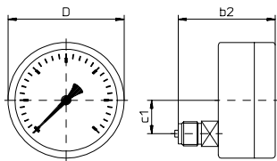
Typ R10.H.1.N...
