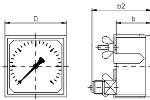
Typ R10.H.2.N...
