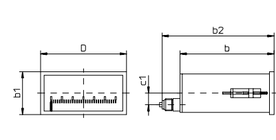
Typ R10.H.2.N...
