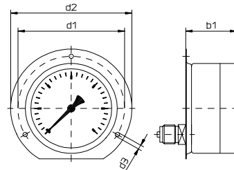
Typ R10.H.3.N...
