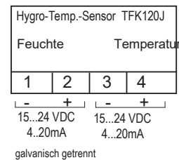
2 Leitersystem
