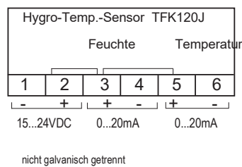
3/4 Leitersystem
