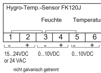
3/4 Leitersystem
