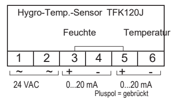
4 Leitersystem (AC-Ausführung)
